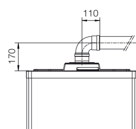
Quota kit orizzontale tiraggio forzato Ø 80
